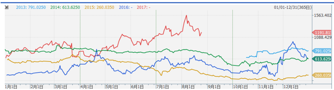
图 3：期货盘面吨钢利润（单位：元/吨）
