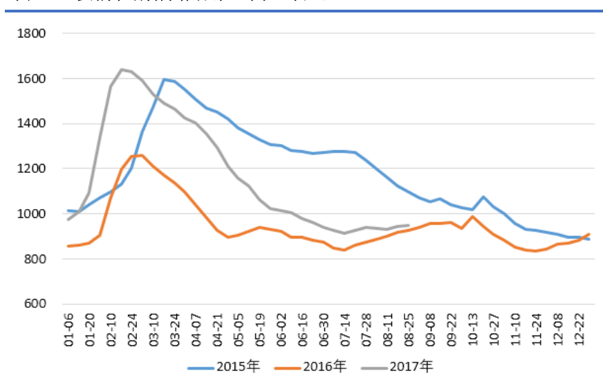
图 2：主要城市钢材库存合计（单位：万吨）
