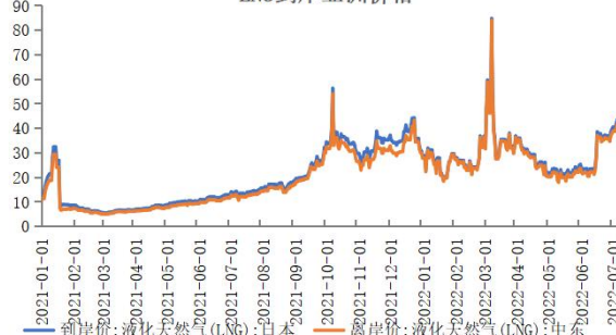
LNG到岸亚洲价格
